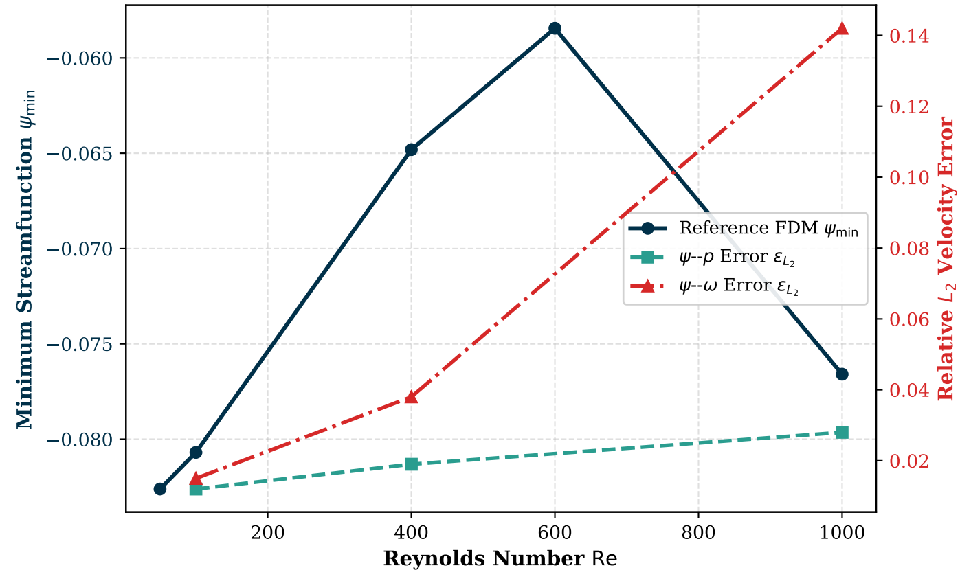
(d) Core Intensity and Formulation Error Scaling
