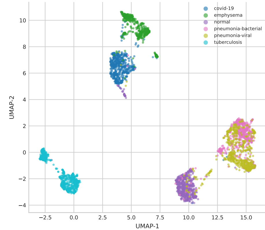
EfficientNet-B0 Silhouette: 0.462
