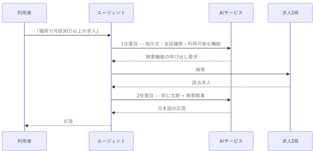
図1 — 利用者が求人を尋ねた場合の処理の流れ
