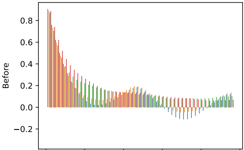
ACF
