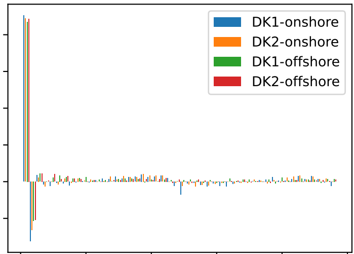
PACF
