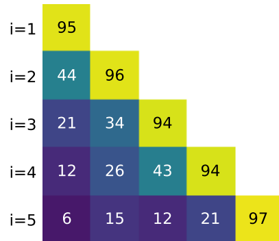
RankExt
