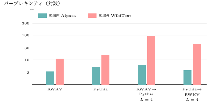
Fig. 6. 領域シフト (文脈 512, 対数軸)。Pythia→RWKV は RWKV→Pythia ( L=4 ) の WikiText perplexity を 93.87 → 45.00 に改善するが, 両親 11.33/16.22 には届かない。同じアダプタが Alpaca では親の近傍にあるため, 長さでなく領域が主要な差である。
