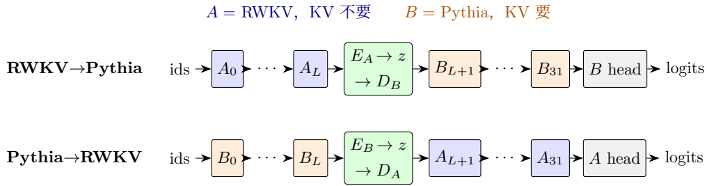
図 2 RWKV→Pythia / Pythia→RWKV キメラモデルの構成。
