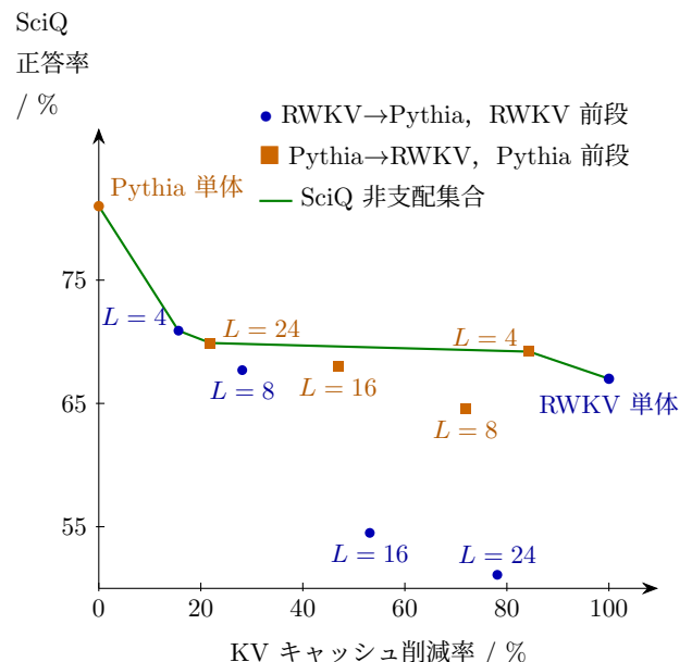
図5 RWKV→Pythia / Pythia→RWKV の SciQ 正答率と KV キャッシュ削減率。緑線は非支配集合に属する構成を結ぶ。
