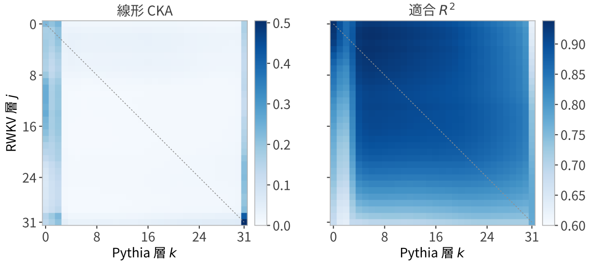
図 3 アダプタを介さない未標準化の残差 h における全 32 \times 32 層の対応. 左は線形 CKA, 右は層ごとの線形写像の適合 R^2 を示す. 破線は同じ番号の層を表し, 二つのパネルで色の尺度が異なる.
