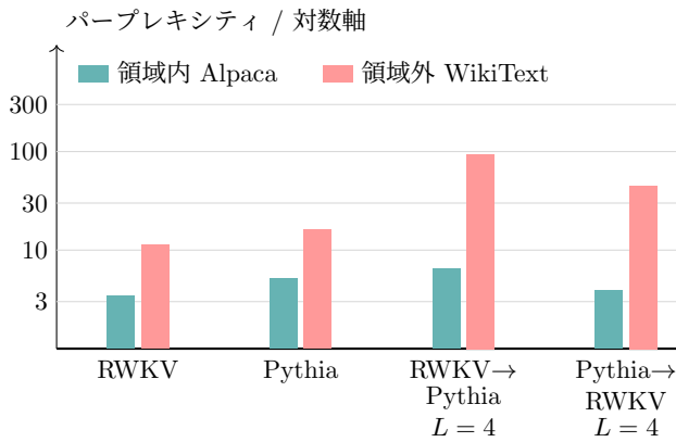
図 6 文脈長 512 における Alpaca と WikiText-103 の perplexity. 縦軸は対数である.
