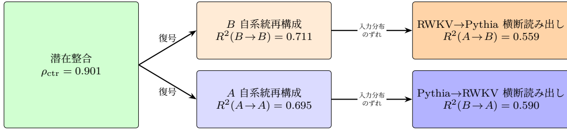
Fig. 3. 共有潜在から両方向の読み出し遷移。橙は復号器 D_B を、青は D_A を通る経路であり、同色の二つは同じ復号器を共有する。高い中心化相関と不完全な自己再構成が共存し、RWKV→Pythia / Pythia→RWKV の横断読み出しは、それぞれ同じ復号器を使う Pythia 自己再構成 / RWKV 自己再構成 を全層で下回る。
