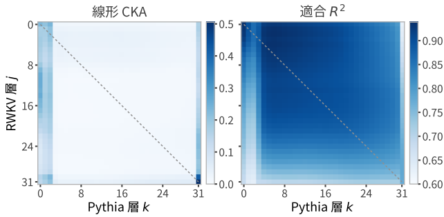
Fig. 2. 生残差の全 32×32 層対応。左：線形 CKA は総じて弱く、高い値は層 0 の行・列と最終層の角に集中する——対角 (破線) は特別でない。右：同じ各ペアへ層別の線形写像をあてはめた適合 R^2 は 0.62–0.94 とほぼ全ペアで高い。二つのパネルの色スケールは異なる。
