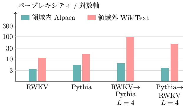
図 6 文脈長 512 における Alpaca と WikiText-103 の perplexity. 縦軸は対数である。
