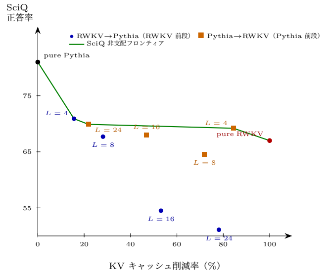
Fig. 5. RWKV→Pythia / Pythia→RWKV の SciQ 正答率と実測 KV 削減率。両経路を含む非支配点は pure Pythia → RWKV→Pythia ( L=4 ) → Pythia→RWKV ( L=24 ) → Pythia→RWKV ( L=4 ) → pure RWKV (緑) となる。これは SciQ 一課題上の事後的フロンティアであり, 経路一般の優越や未知課題への汎化を意味しない。
