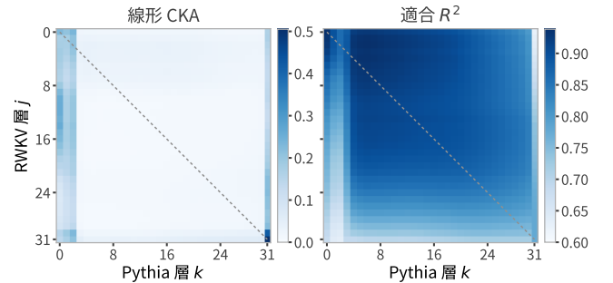
Fig. 2. 生残差の全 32 \times 32 層対応。左: 線形 CKA は総じて弱く、高い値は層 0 の行・列と最終層の角に集中する——対角 (破線) は特別でない。右: 同じ各ペアへ層別の線形写像をあてはめた適合 R^2 は 0.62–0.94 とほぼ全ペアで高い。二つのパネルの色スケールは異なる。
