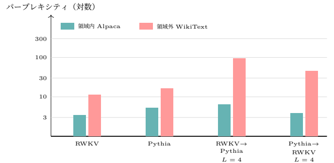
Fig. 6. 領域シフト (文脈 512, 対数軸)。Pythia→RWKV は RWKV→Pythia ( L=4 ) の WikiText perplexity を 93.87 \rightarrow 45.00 に改善するが, 両親 11.33/16.22 には届かない。同じアダプタが Alpaca では親の近傍にあるため, 長さでなく領域が主要な差である。
