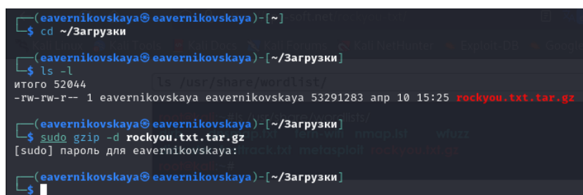
Рис. 3.2: Распаковка архива со списком паролей
