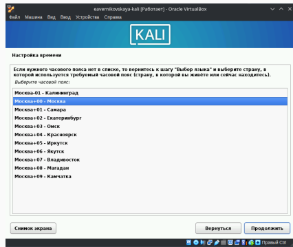
Рис. 15: Настройка времени
