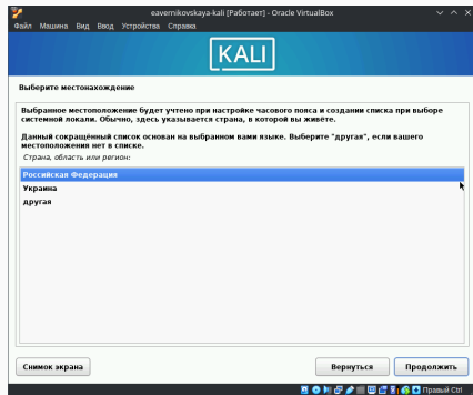
Рис. 7: Выбор местонахождения
