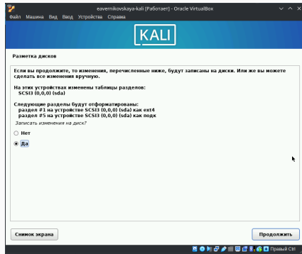
Рис. 20: Разметка дисков (5)
