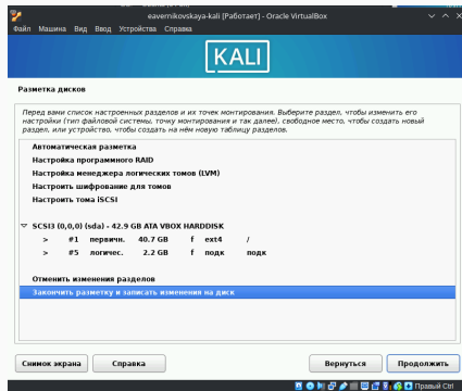
Рис. 19: Разметка дисков (4)
