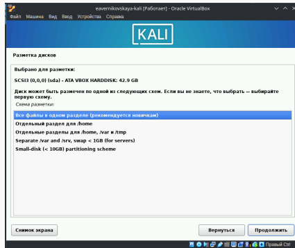
Рис. 18: Разметка дисков (3)
