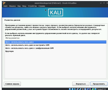
Рис. 16: Разметка дисков (1)
