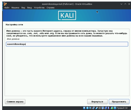
Рис. 11: Настройка сети (2)
