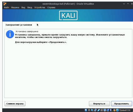
Рис. 24: Завершение установки
