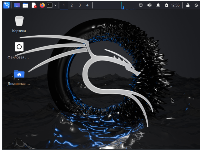
Рис. 26: Kali Linux :)
