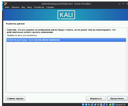
Рис. 17: Разметка дисков (2)
