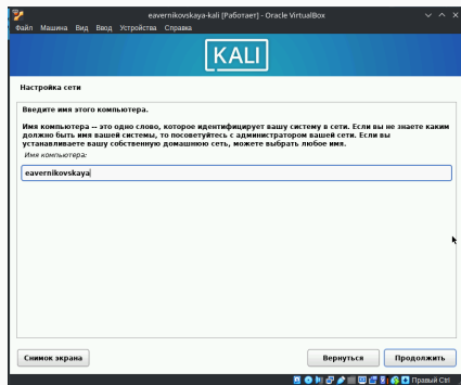
Рис. 10: Настройка сети (1)
