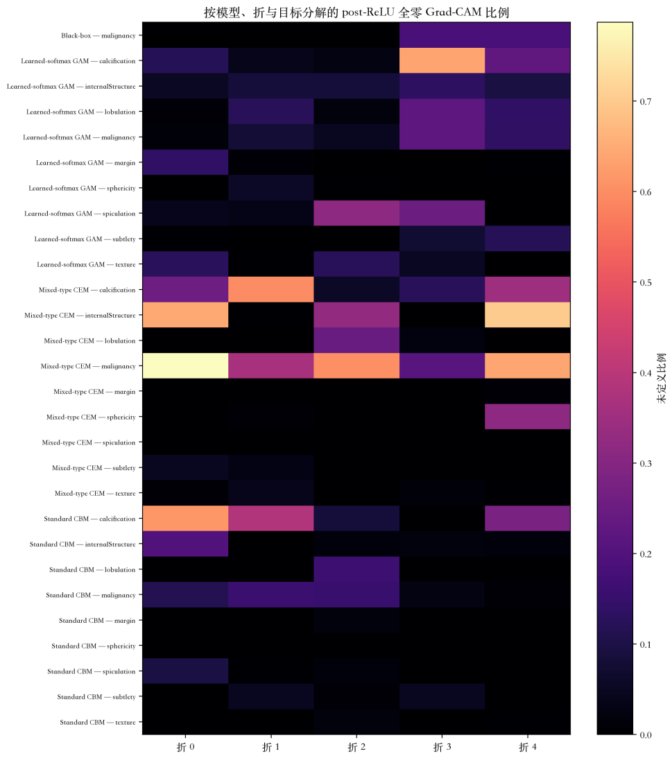
RPT-F07. 按模型、折和目标分解的 post-ReLU 全零 Grad-CAM 比例。
