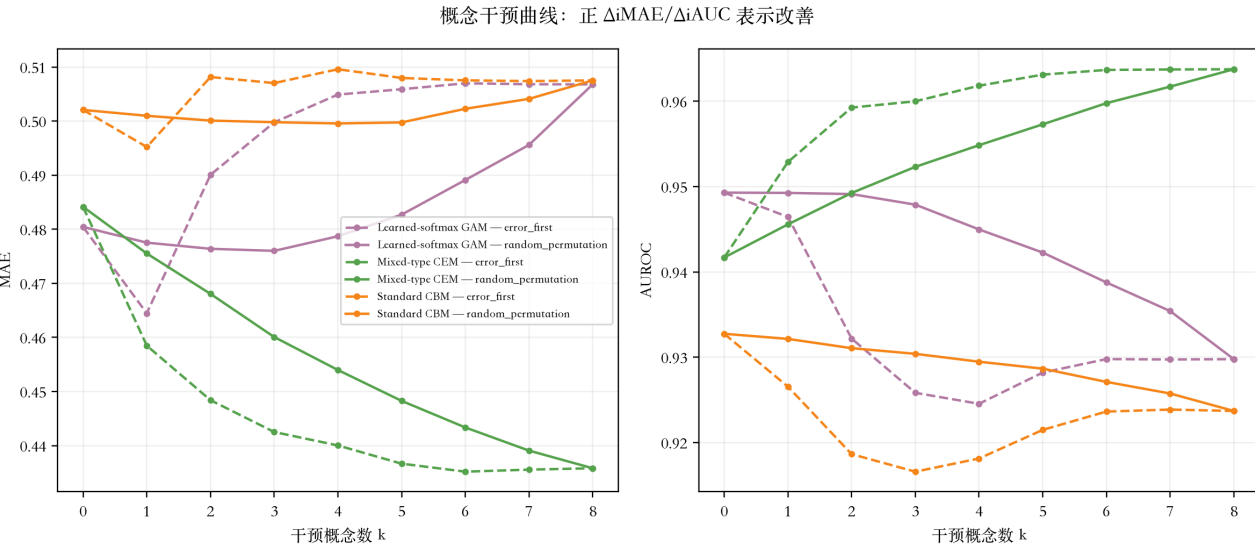
RPT-F12. 随机顺序与 error-first 顺序下的 k=0...8 概念干预曲线。
