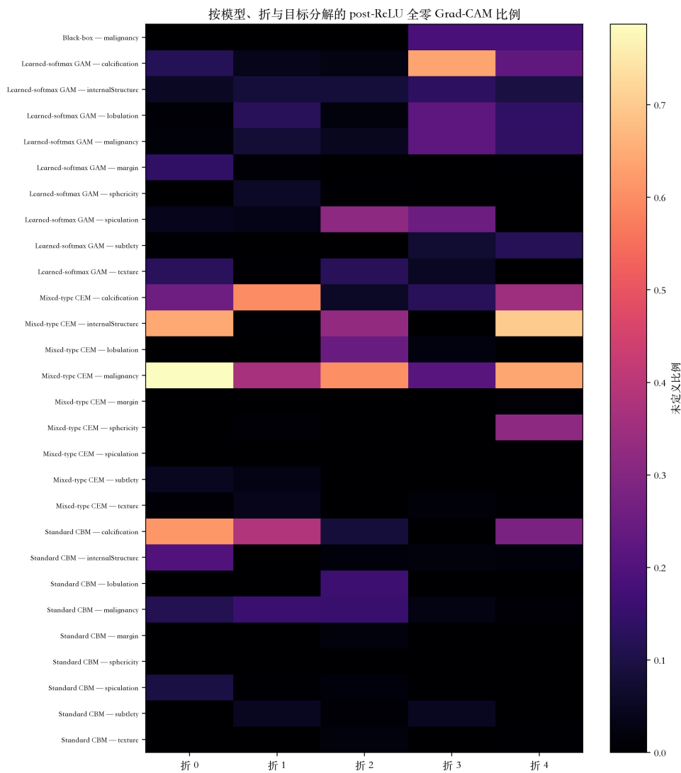
RPT-F07. 按模型、折和目标分解的 post-ReLU 全零 Grad-CAM 比例。
