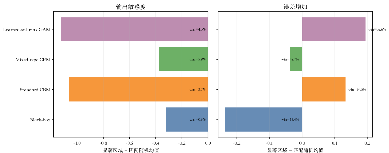
RPT-F08. output_sensitivity 与 error_increase 相对匹配随机遮挡的空间忠实度。
