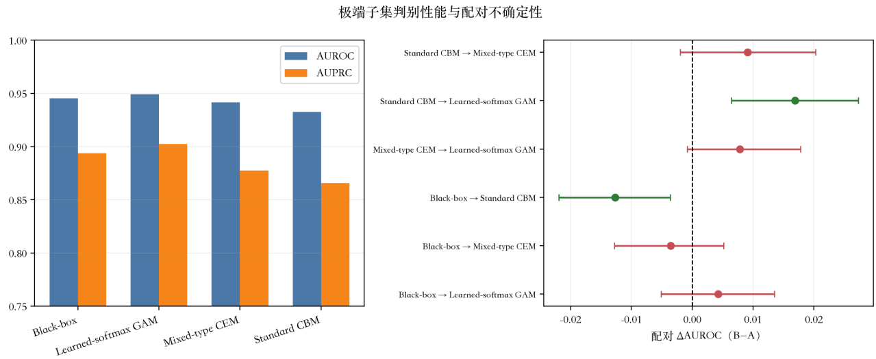
RPT-F06. 极端任务 AUROC/AUPRC 与六组配对 Delta-AUROC。
