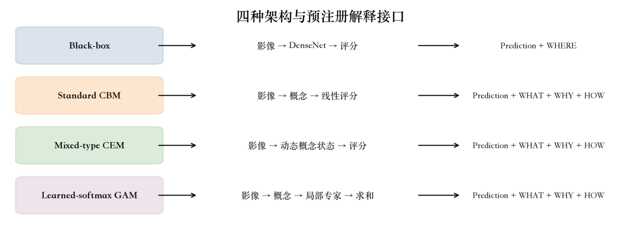
RPT-F03. 四种模型架构及其预注册解释接口。
