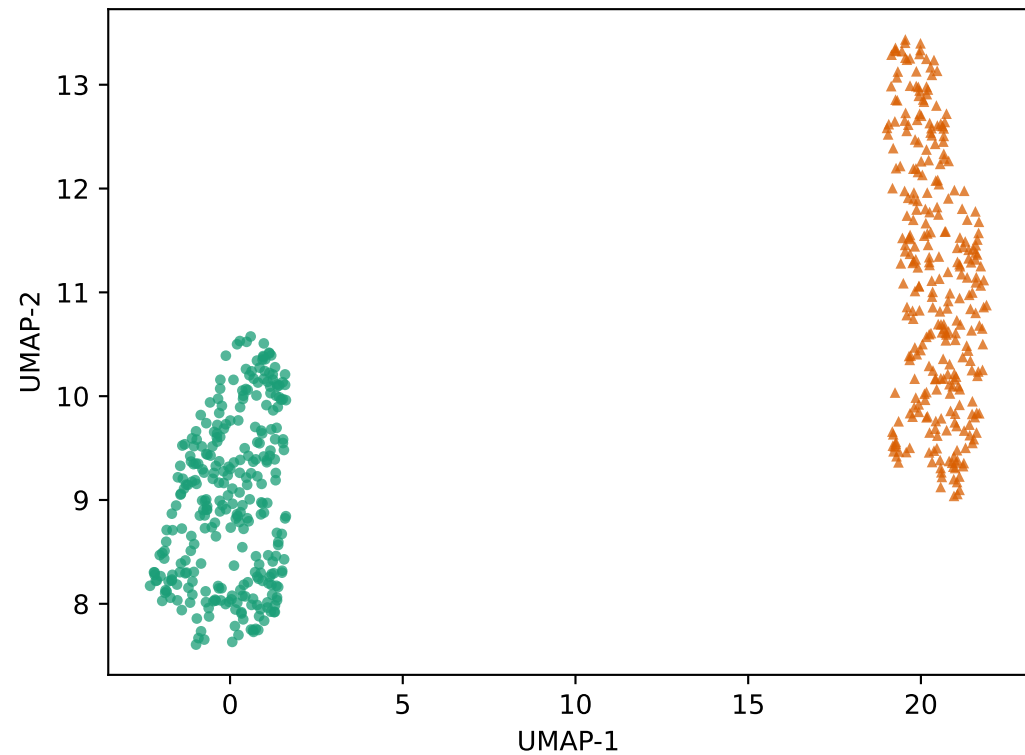
WavLM Layer 9
