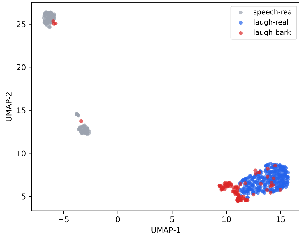
WavLM Layer 9
