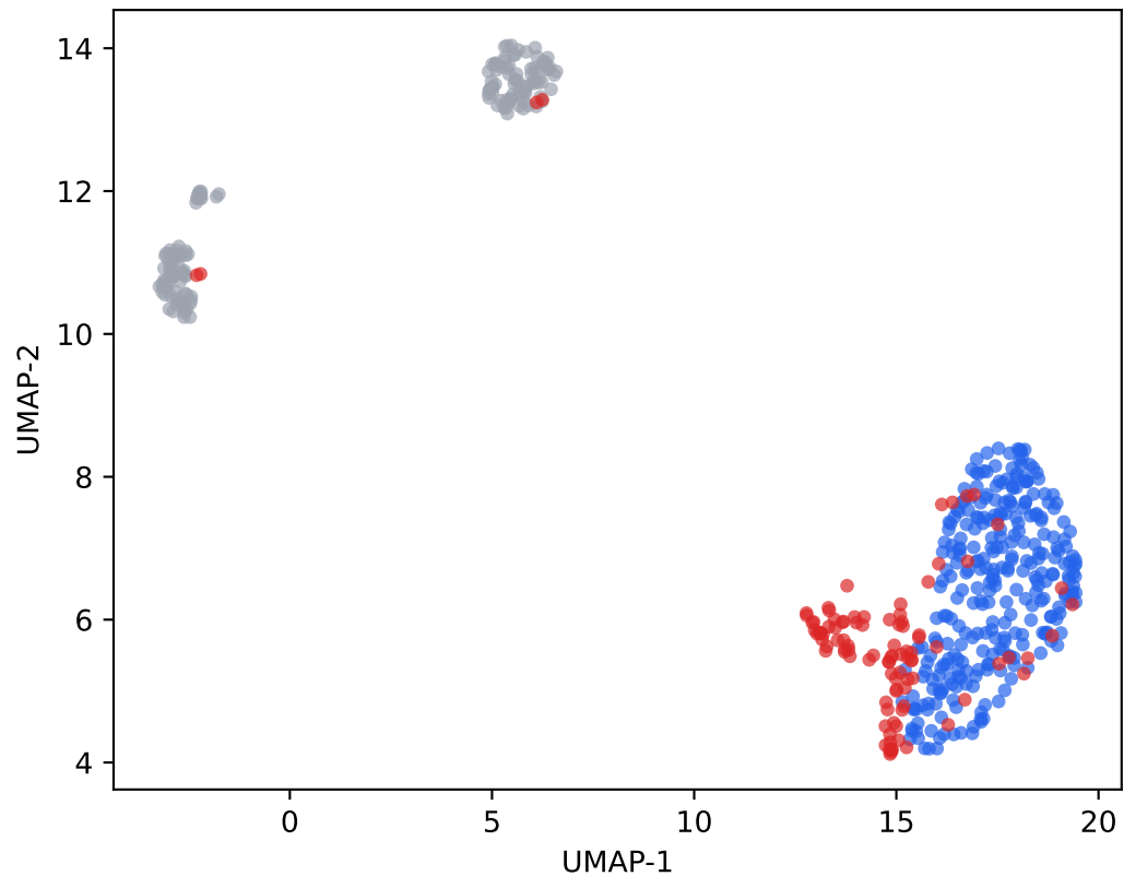
WavLM Layer 12
