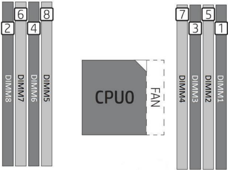
図1 DIMM装着順。図の数字は装着する順番で、DIMM番号とは異なる。HP QuickSpecs v62 p21の部分図 [R1]。現在の個別DIMM使用位置は未確定。
