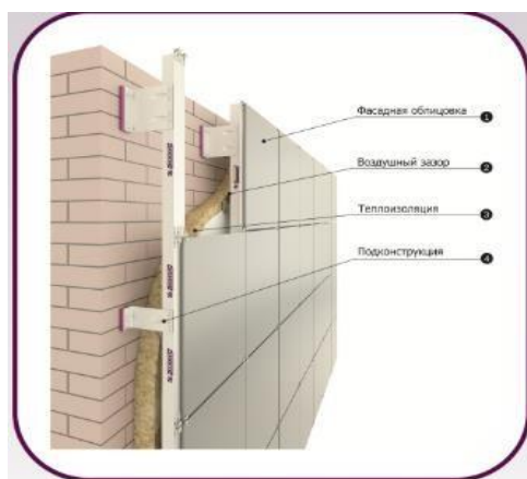
Рисунок 2.9. Схема навесного вентилируемого фасада
