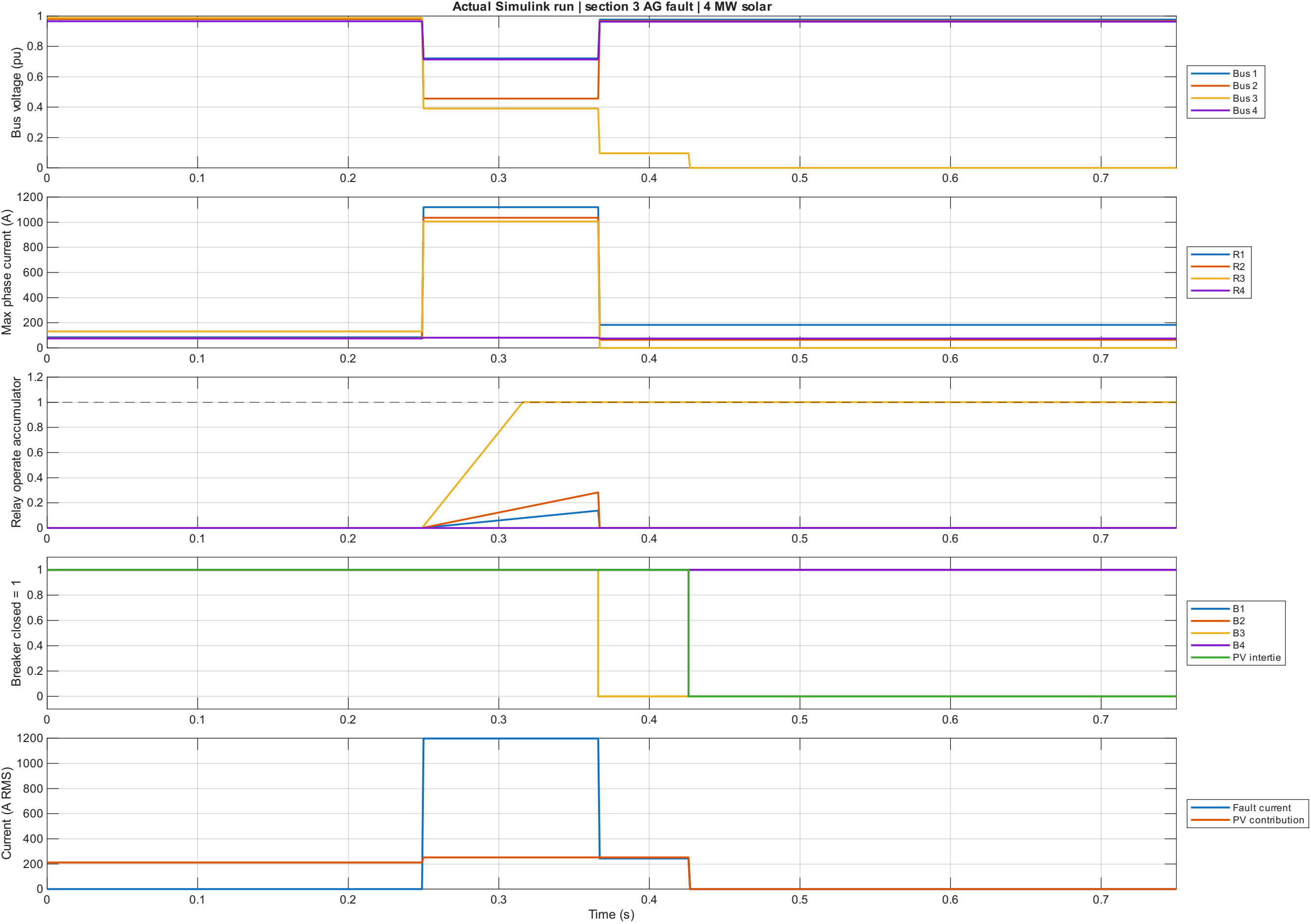
Actual Simulink run | section 3 AG fault | 4 MW solar
