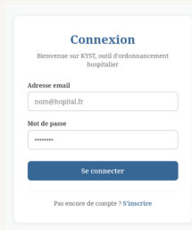
Connexion
