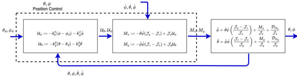
Figura 2: Malhas internas de posição de roll e pitch .
