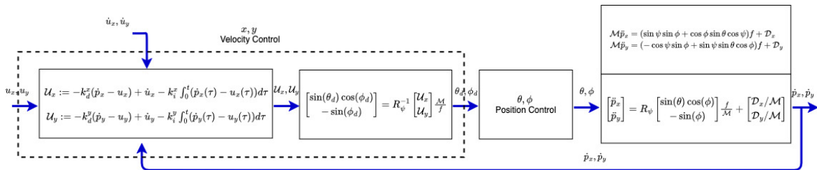
Figura 3: Malha interna de velocidade (x, y) . Fonte: [Peixoto (2025)].
