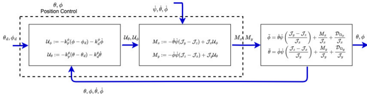
Figura 2: Malhas internas de posição de roll e pitch. Fonte: [Peixoto (2025)].
