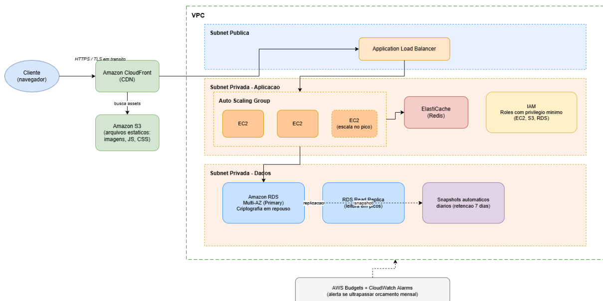
Arquitetura AWS - Loja Virtual com Picos na Black Friday (Cenário A)
