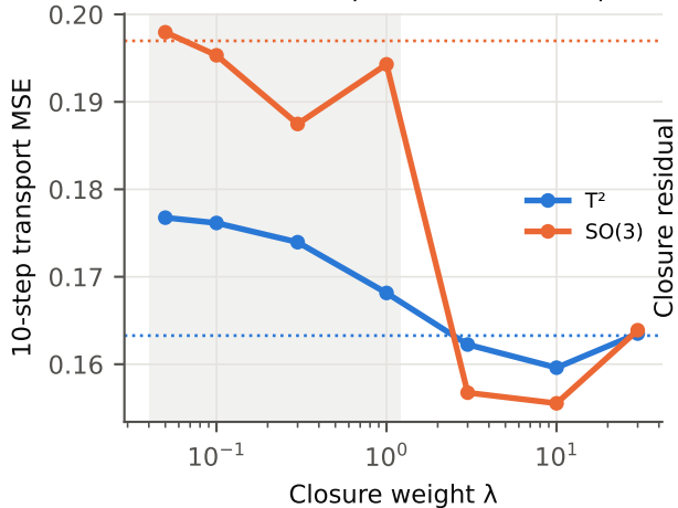
Validation transport (dotted: +Comp.)
