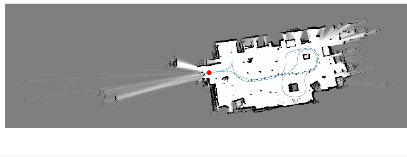
LiDAR · scan-to-map · ICP
