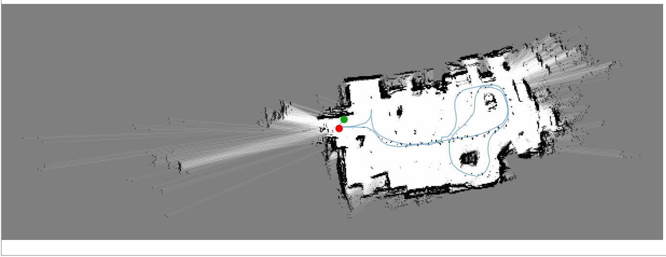
LiDAR · scan-to-submap · ICP
