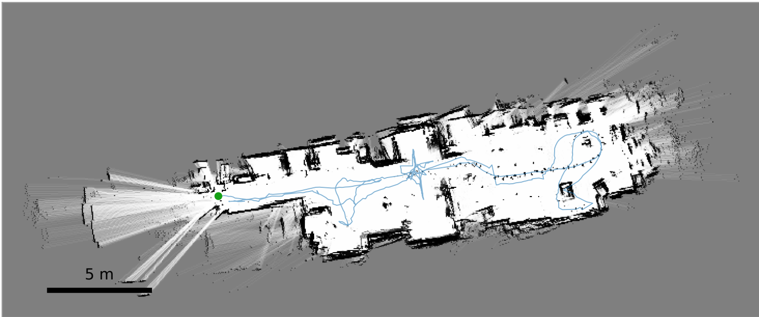
Two-room lab — Visual VO + LiDAR-B&B verify
