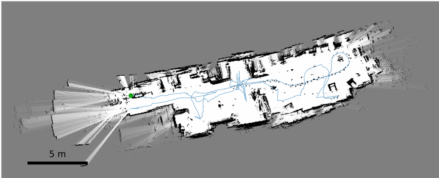
Two-room lab — Visual VO + LiDAR-ICP verify
