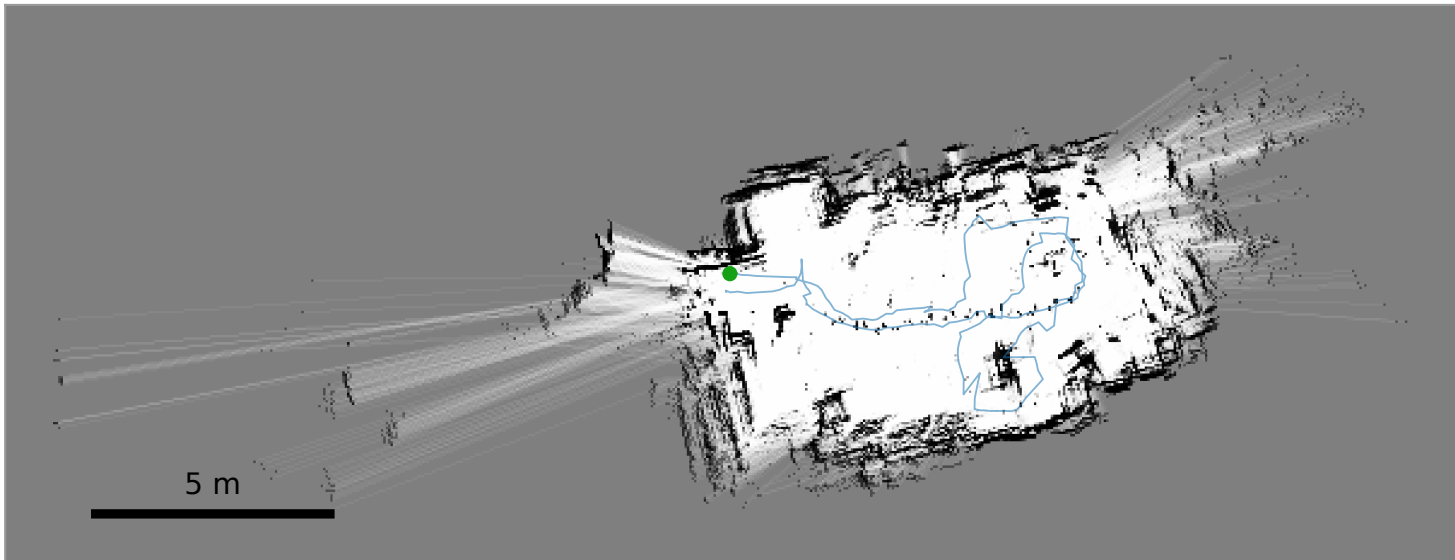
Single-room lab — Visual VO + LiDAR-ICP verify
