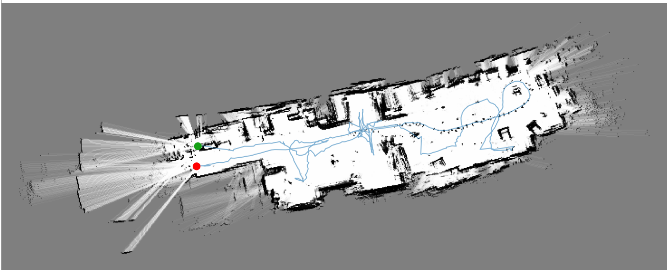
Visual VO + LiDAR-ICP verify
