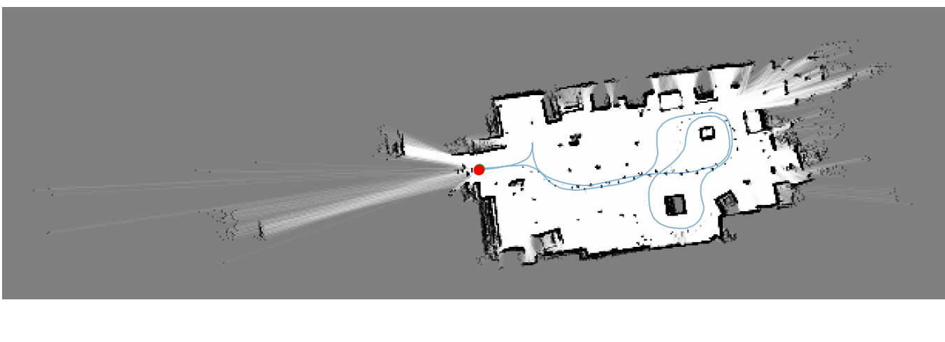
LiDAR · scan-to-map · B&B
