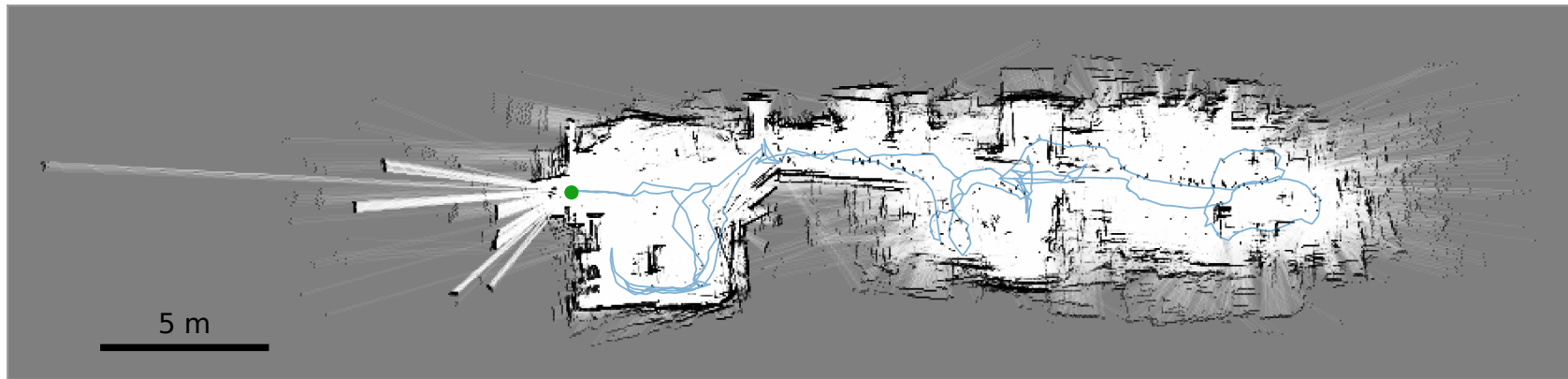
lab_hybrid_3 — Visual VO + LiDAR-B&B verify
