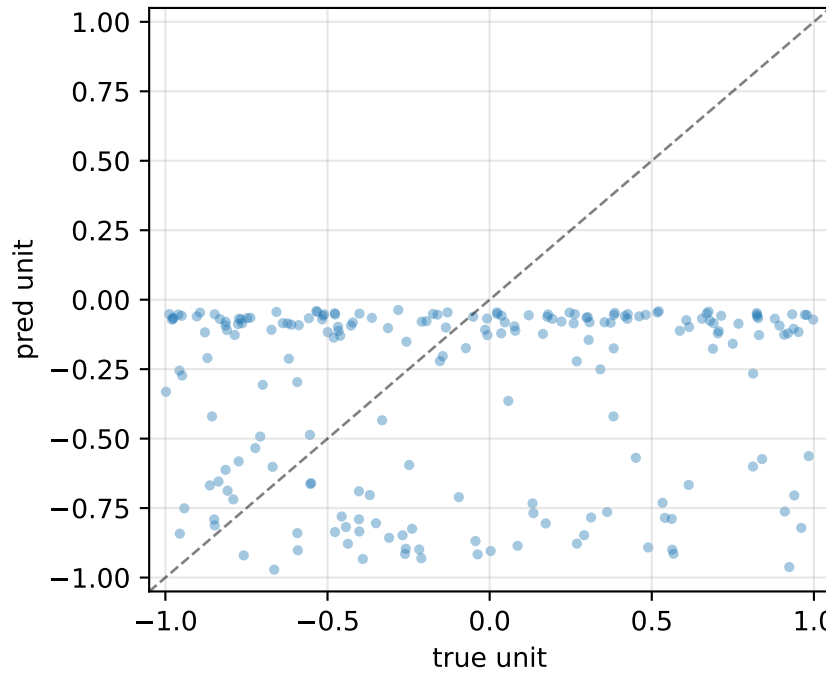
gNaTs2_tbar_NaTs2_t_somatic R^2=-0.78 MSE=0.595
