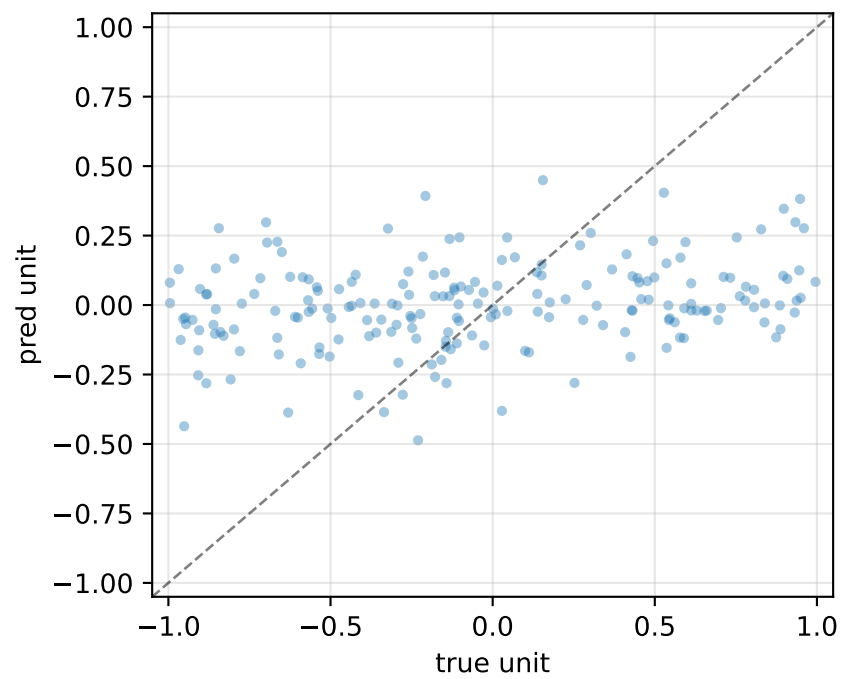
gK_Tstbar_K_Tst_axonal R^2=-0.03 MSE=0.336
