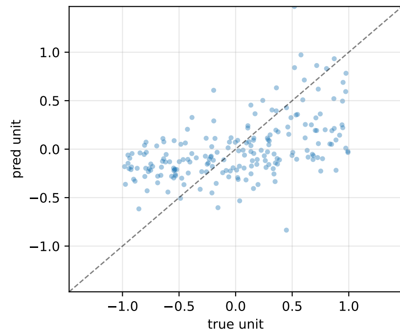
glhbar_lh_dend R^2=+0.51 MSE=0.165
