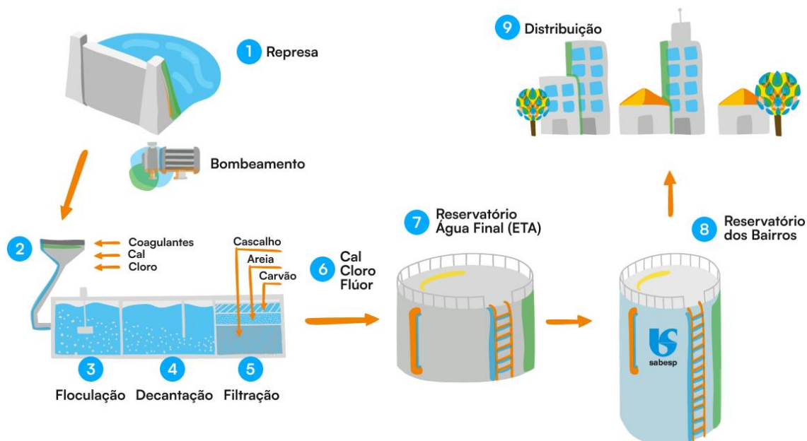
FIGURA 4 – INFOGRÁFICO DO PROCESSO DE TRATAMENTO DE ÁGUA PELA SABESP NAS ESTAÇÕES DE TRATAMENTO DE ÁGUA (ETAS)
