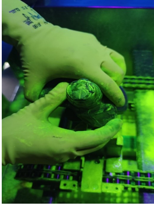
Şekil 18.1. UV-A altında floresan manyetik parçacık muayenesinden saha görüntüsü.
