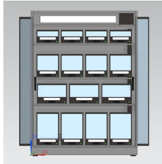
b) Malzeme dolabı tasarımı
