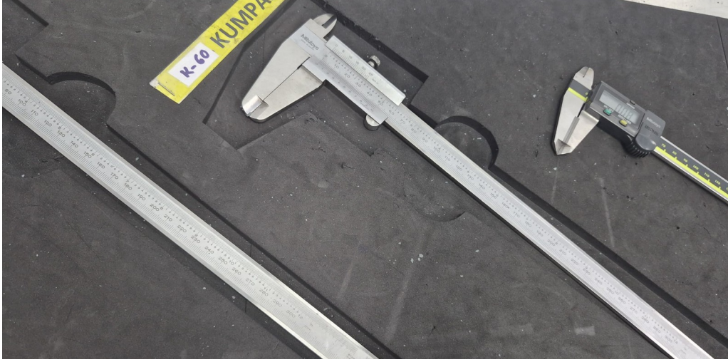
Şekil 26.1. Kalite kontrol bölümündeki kumpas ve ölçüm aletlerinin yerleşimi (staj fotoğrafı).
