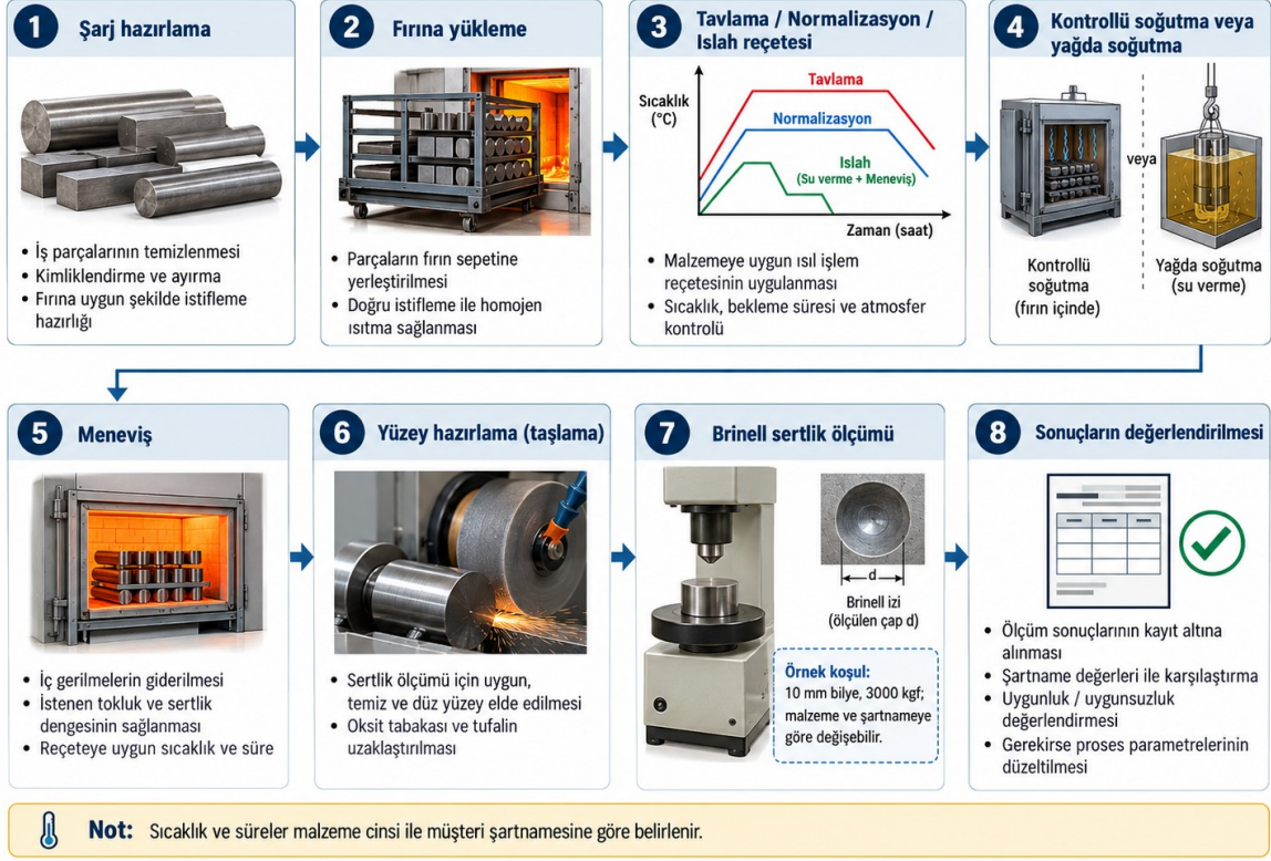
Şekil 16.1. Isıl işlem ve Brinell sertlik kontrolünün şematik gösterimi.
