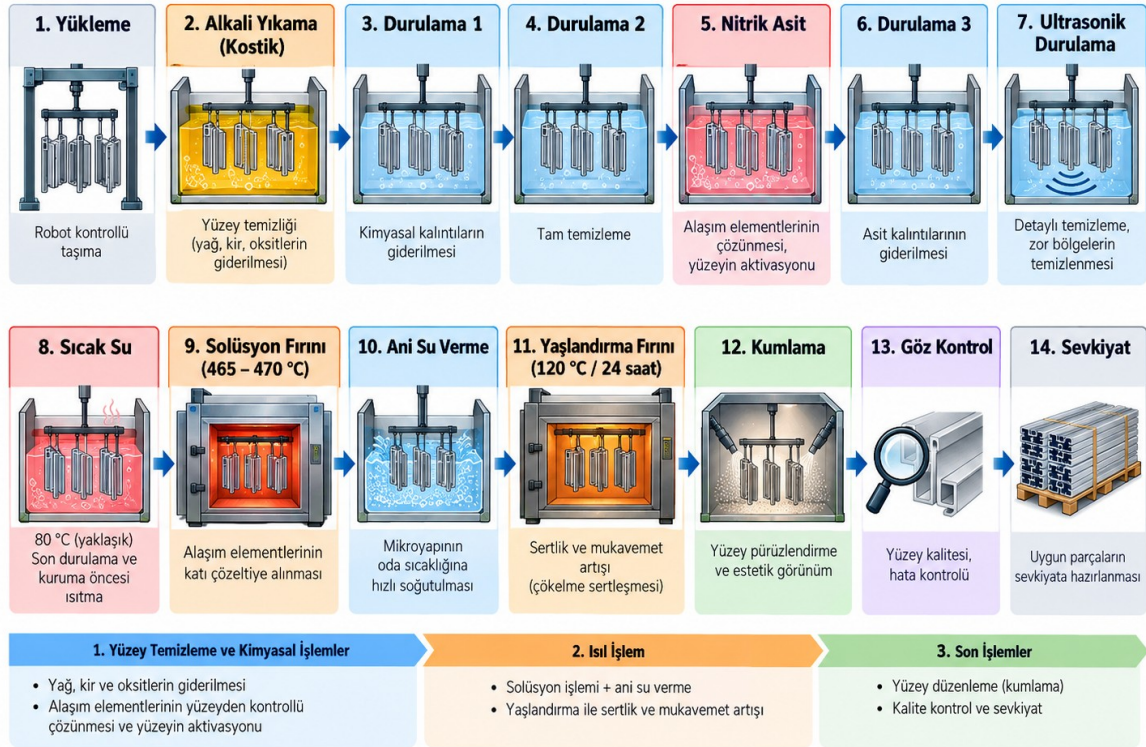
Şekil 17.1. Alüminyum yıkama, solüsyona alma ve yaşlandırma hattının şematik gösterimi.
