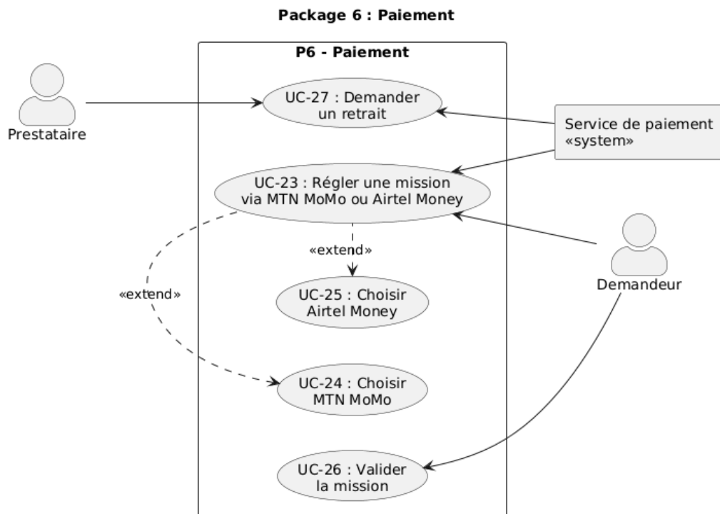
Figure 10 : Diagramme de cas d'utilisation - P6 : Paiement
