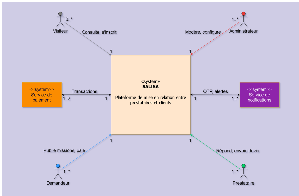
Figure 4 : Diagramme de contexte statique de « SALISA »
