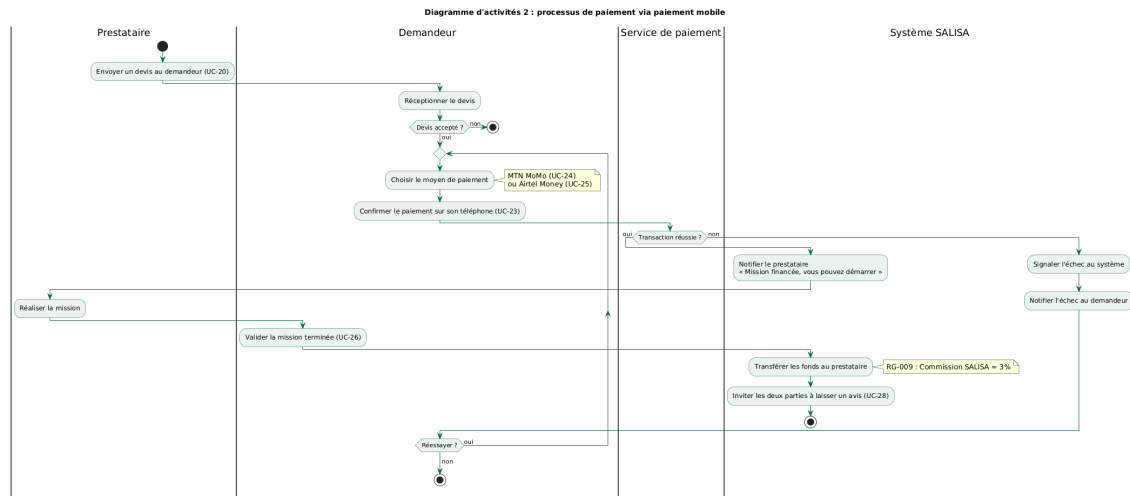
Figure 18 : Diagramme d'activités - processus de paiement mobile
