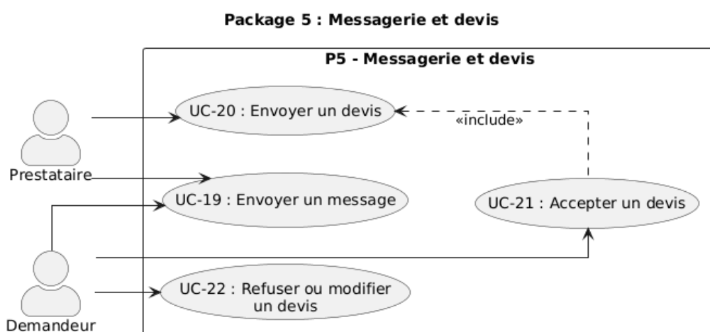
Figure 9 : Diagramme de cas d'utilisation - P5 : Messagerie et devis
