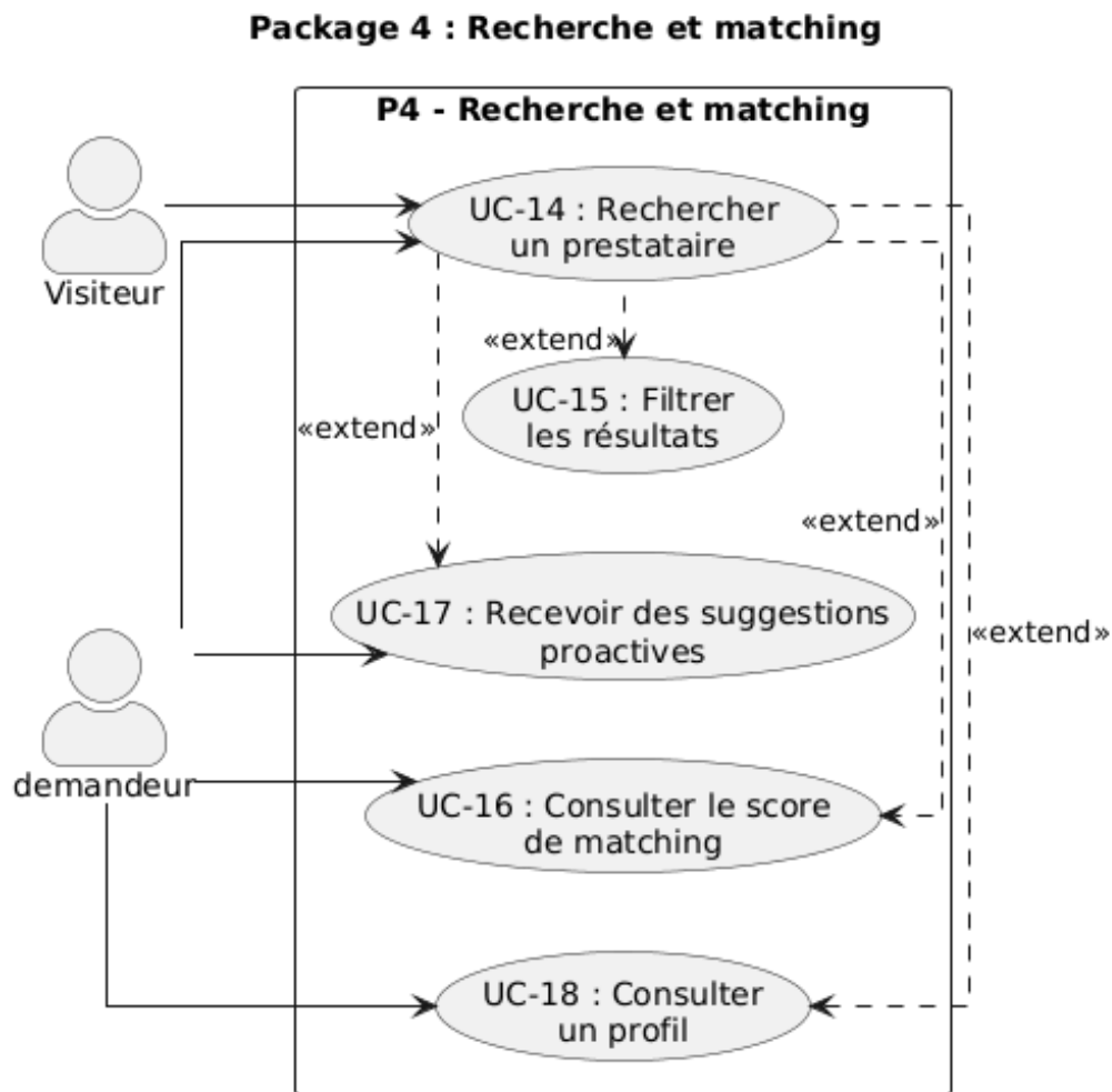
Figure 8 : Diagramme de cas d'utilisation - P4 : Recherche et matching
