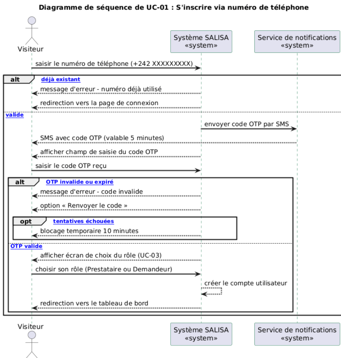
Figure 15 : Diagramme de séquence - inscription via numéro de téléphone (UC-01)
