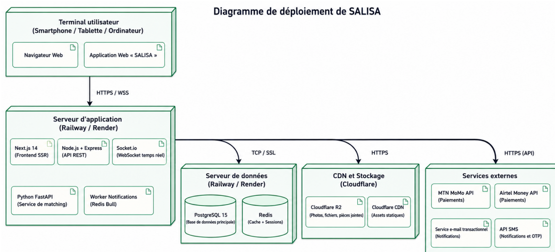
Figure 22 : Diagramme de déploiement de SALISA
