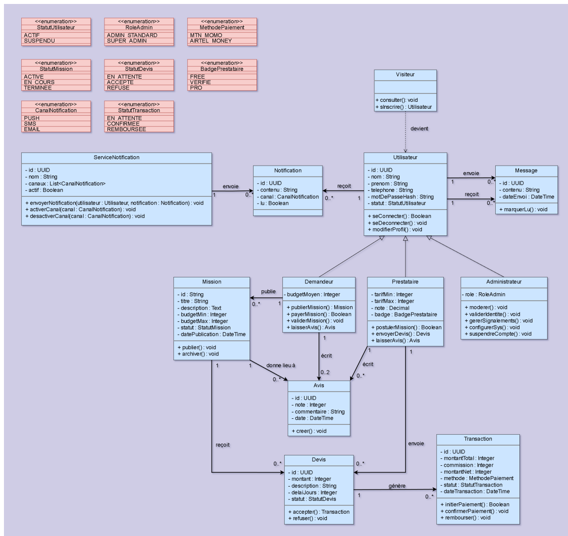
Figure 20 : Diagramme de classes du système « SALISA »
