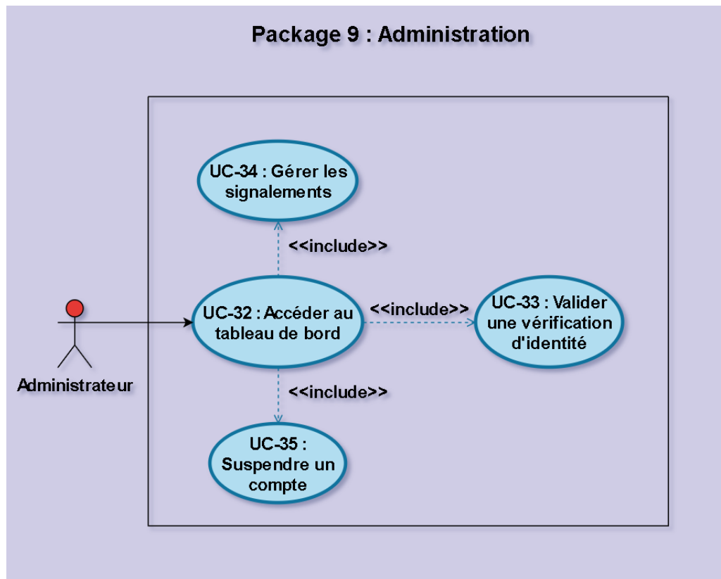
Figure 14 : Diagramme de cas d'utilisation - Package 9 : Administration
