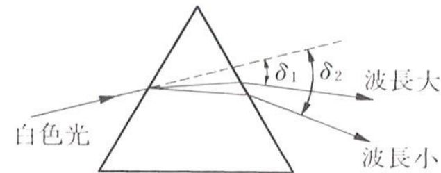
図 2.5 プリズムによる分光
