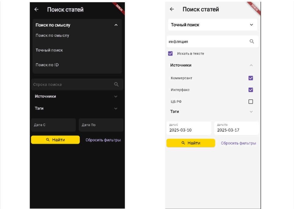
Рисунок 5. Страница поиска по статьям
