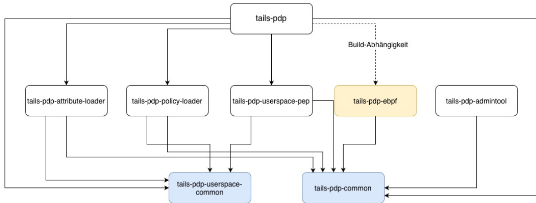
Abbildung 2: Interne Abhängigkeiten der Rust-Crates. Durchgezogene Pfeile kennzeichnen reguläre Cargo-Abhängigkeiten, der gestrichelte Pfeil die Build-Abhängigkeit zur Erzeugung des eingebetteten eBPF-Artefakts. Pfeile zeigen von der abhängigen Crate zur verwendeten Crate. Externe Abhängigkeiten sind nicht dargestellt. Eigene Darstellung.
