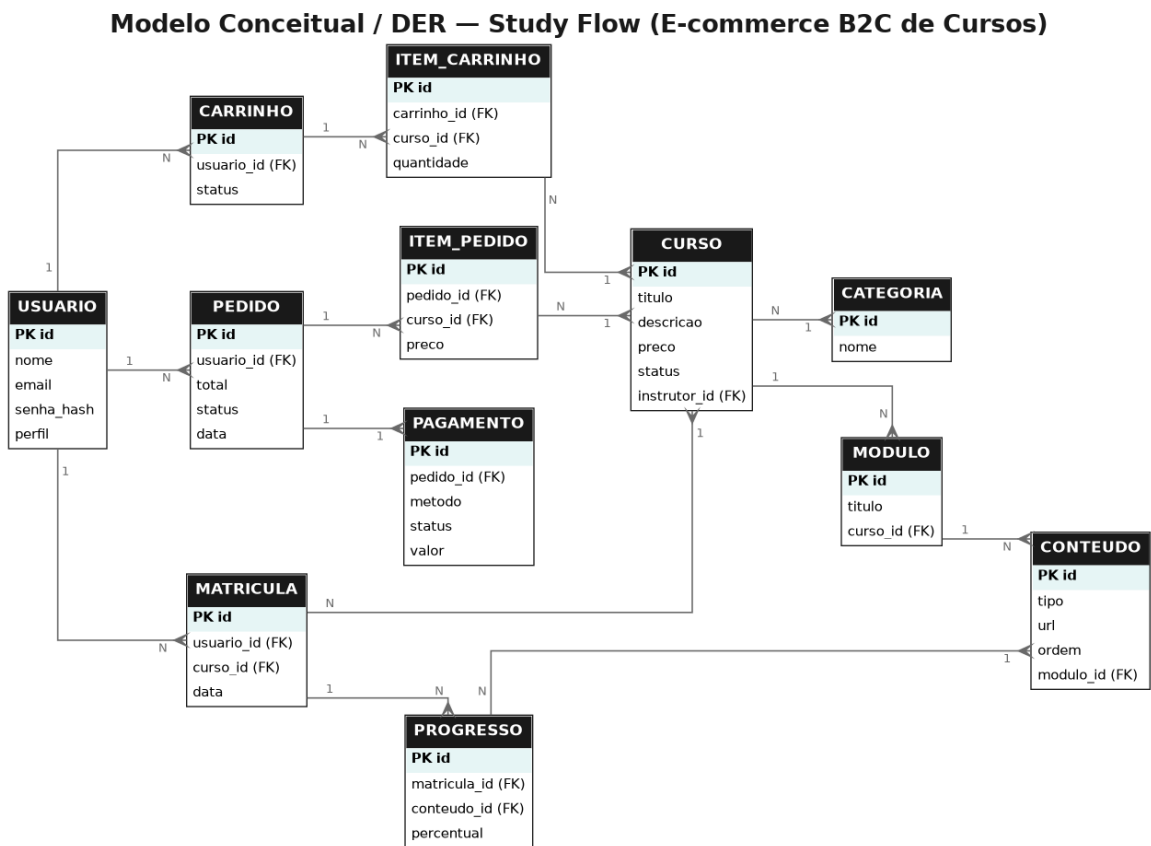
Figura 1 — Modelo conceitual/DER proposto para o Study Flow.
