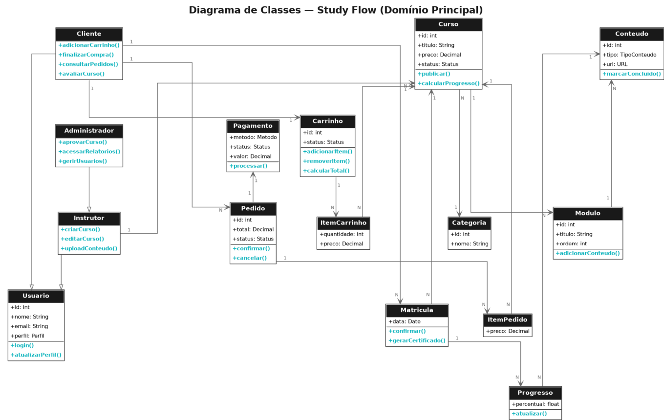
Figura 2 — Diagrama de classes simplificado do domínio principal do Study Flow.
