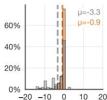
GPT-4o
