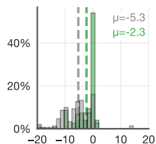
Gemma 3 27B
