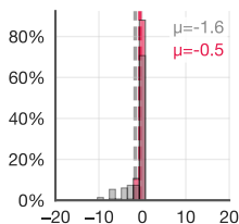
Gemini 2.0 Flash
