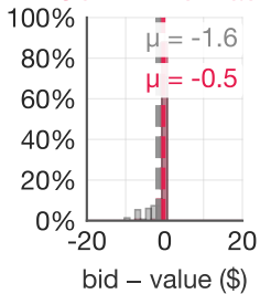
Gemini 2.0 Flash
