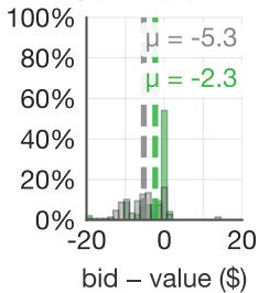
Gemma 3 27B
