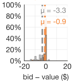
GPT-4o
