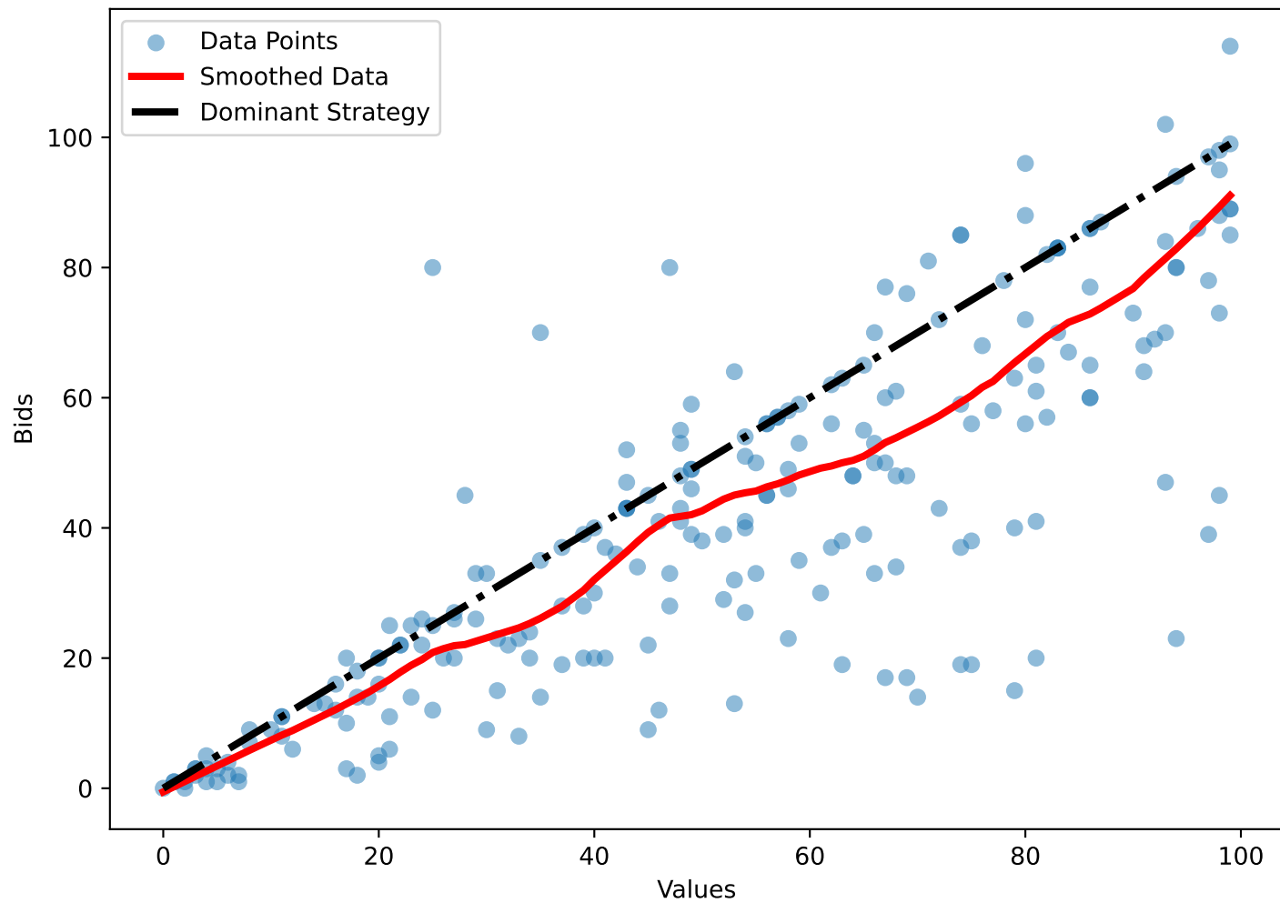
Bids vs. Values (Private Values - SPSB)
