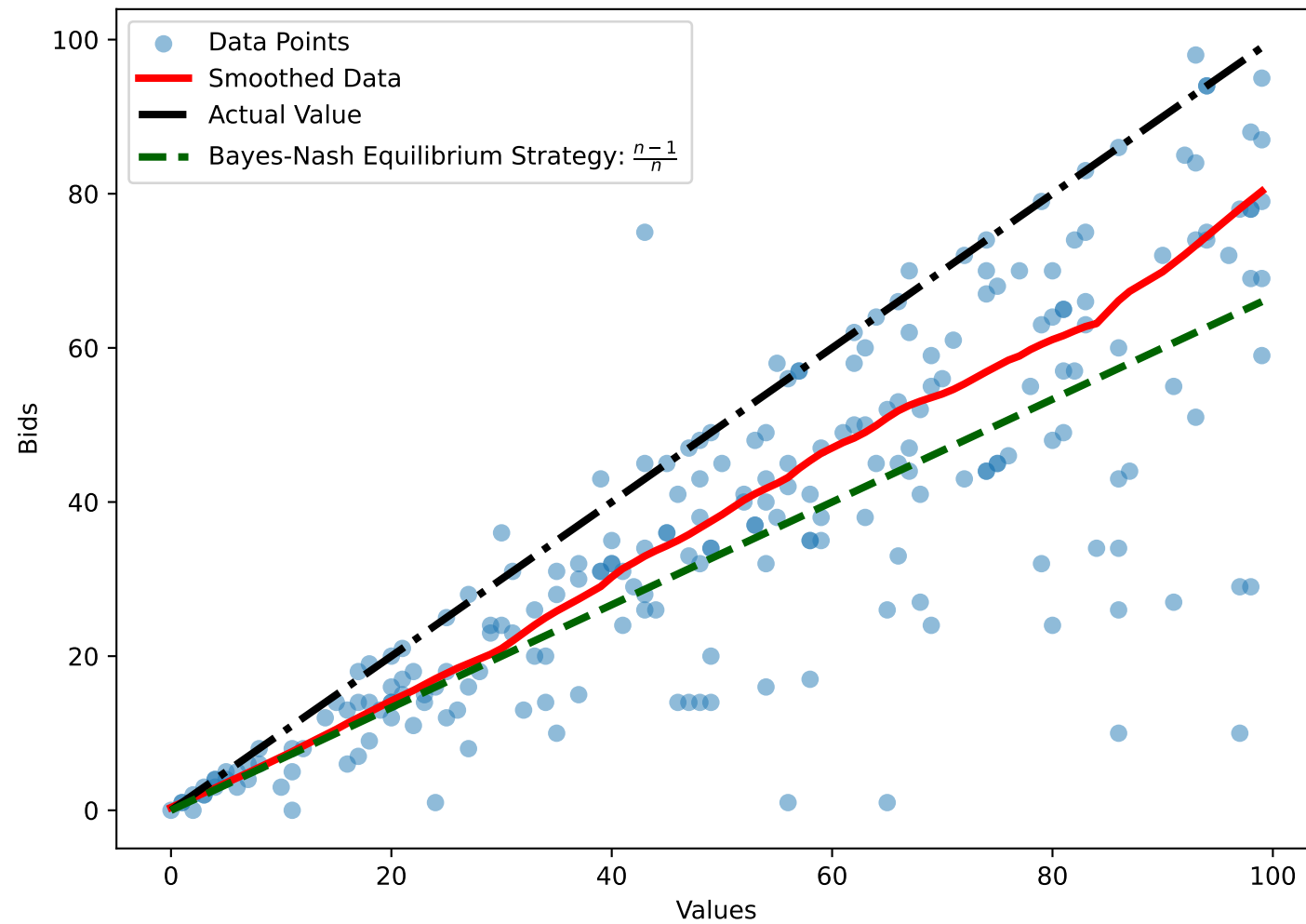
Bids vs. Values (Private Values - FPSB)
