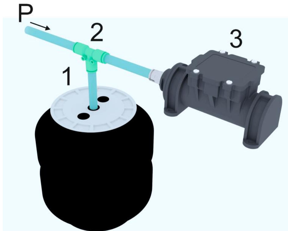
1 – Пневмоподушка, 2 – Фитинг-тройник, 3 – Блок измерительный eCargosens Air, P – Подача давления
