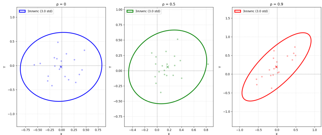
Рис 1. Пример графика для функции plot_subplots_ellipses .
