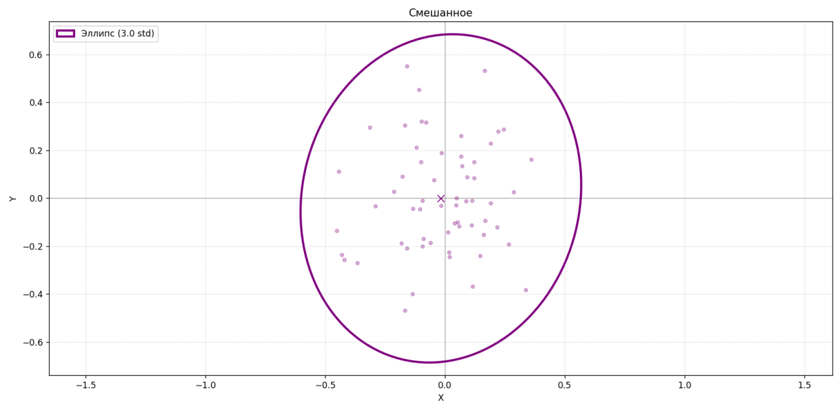
Рис 6. Эллипс рассеяния для смеси распределений при размере выборки 60
