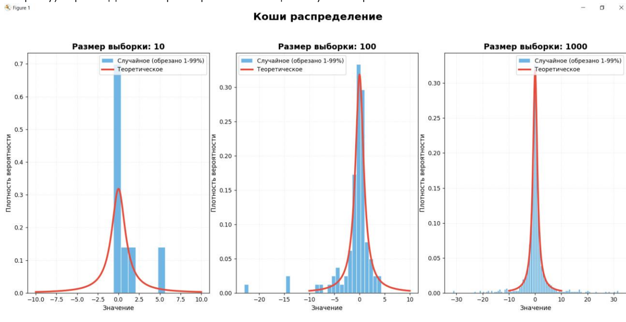
Рис 6. Гистограммы для распределения Коши
