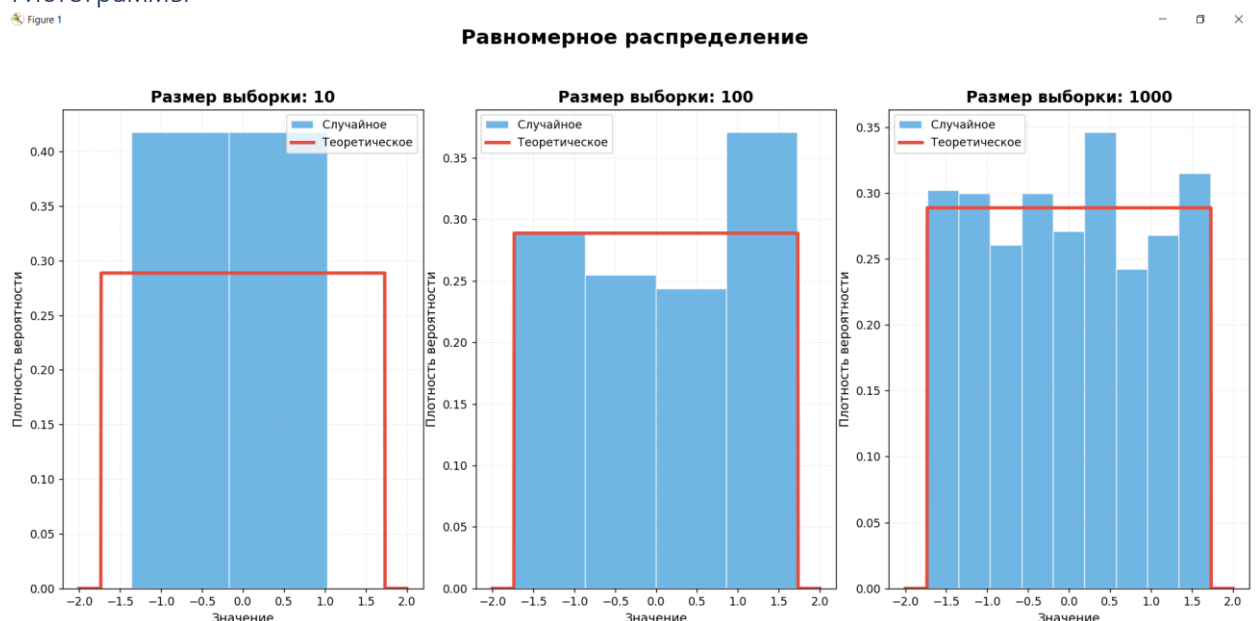
Рис 12. Гистограммы для равномерного распределения
