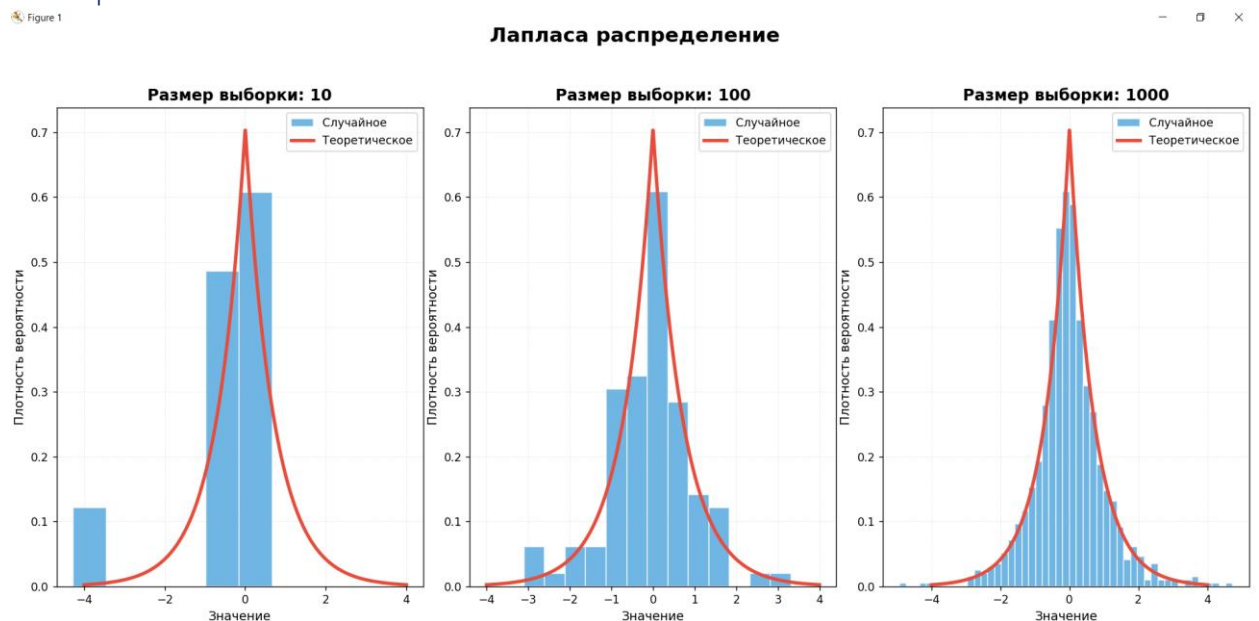
Рис 8. Гистограммы для распределения Лапласа
