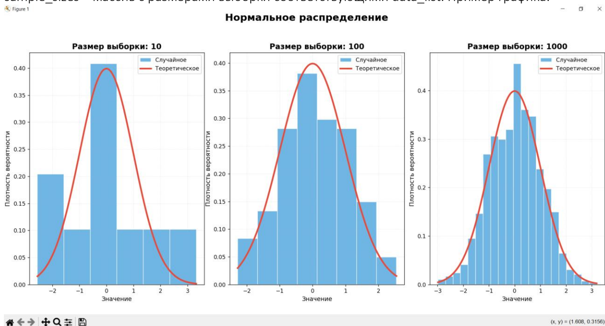
Рис 1. Пример графика для функции paint_distribution
