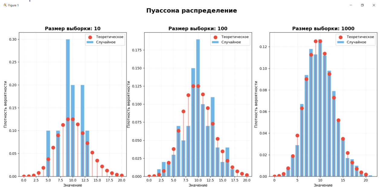
Рис 10. Гистограммы для распределения Пуассона
