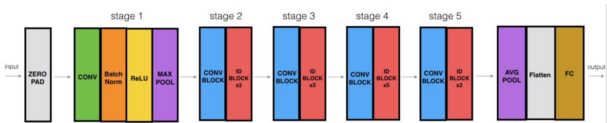
2.12 kiến trúc resnet
