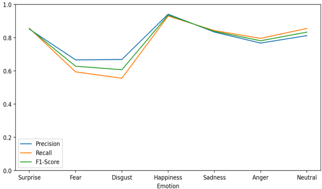
4.6 biểu đồ biểu diễn các thông số dựa trên cảm xúc
