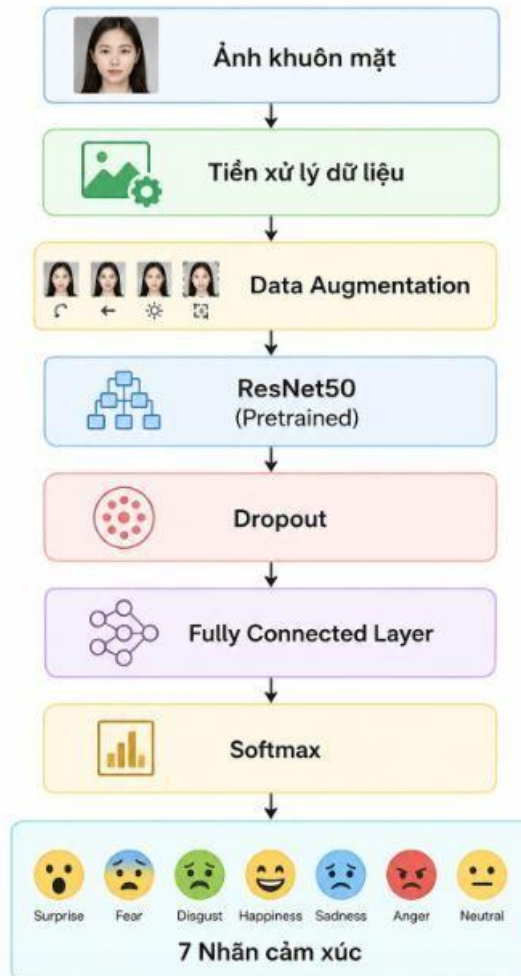
1.1 Các bước nhận diện cảm xúc
