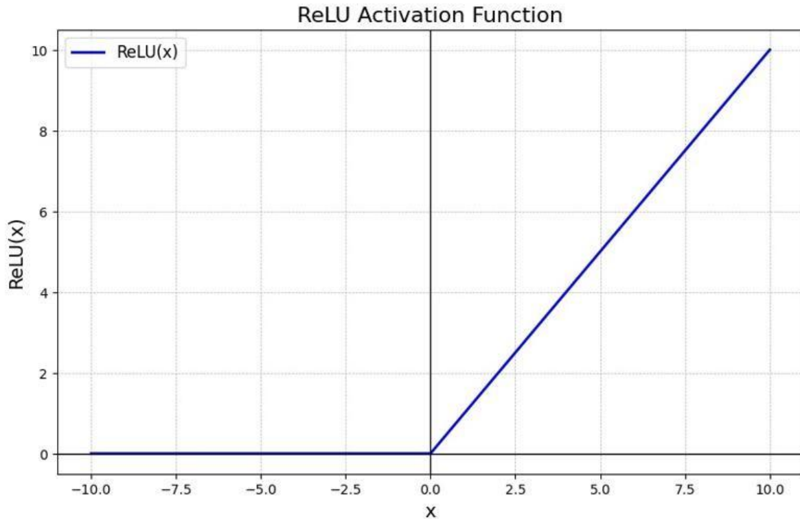
2.4 hàm relu
