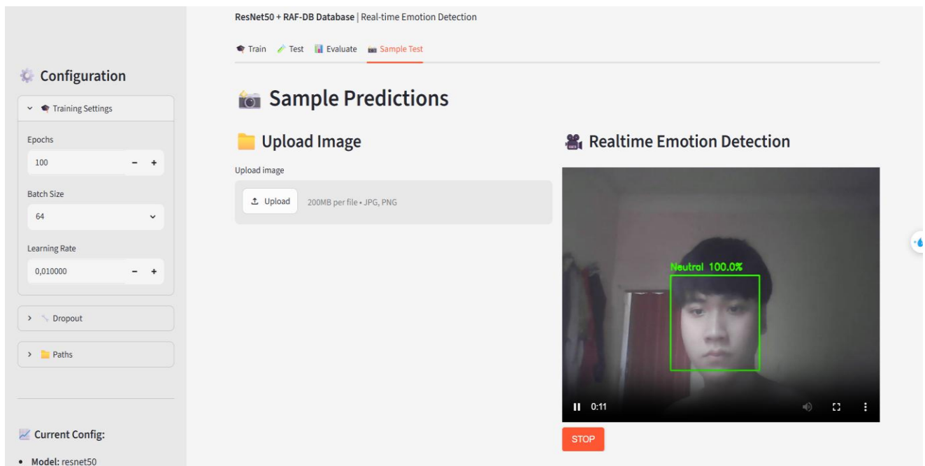
4.11 Chạy realtime nhận diện cảm xúc theo thời gian thực
