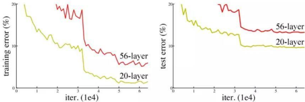
2.9 Biểu đồ hiện thị hiện tượng vanishing gradient với các lớp sâu
